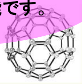
フラレンの構造
