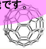
フラーレンの構造
