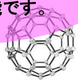
フラーレンの構造
