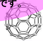
フラレンの構造
