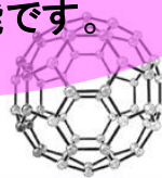
フラレンの構造
