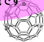
フラレンの構造
