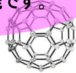
フラーレンの構造
